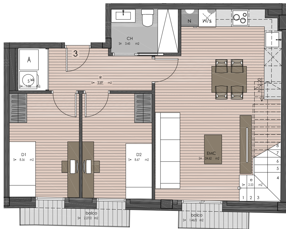
PLANTA TERCERA
