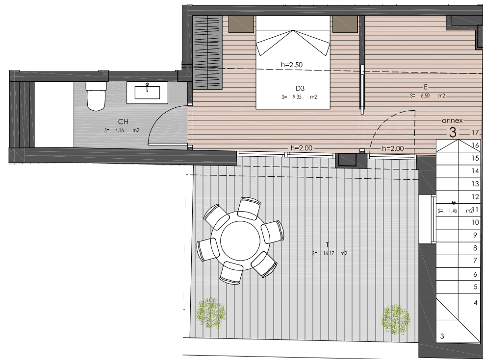
PLANTA SOTACOBERTA
