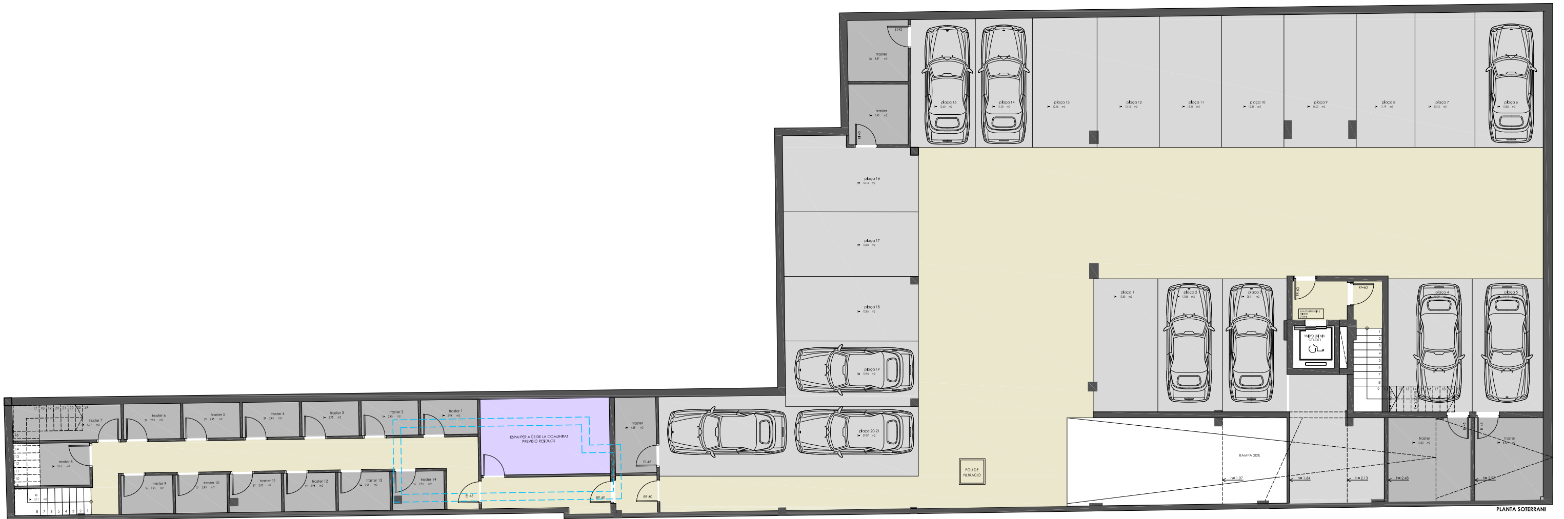
PLANTA SOTERRANI
