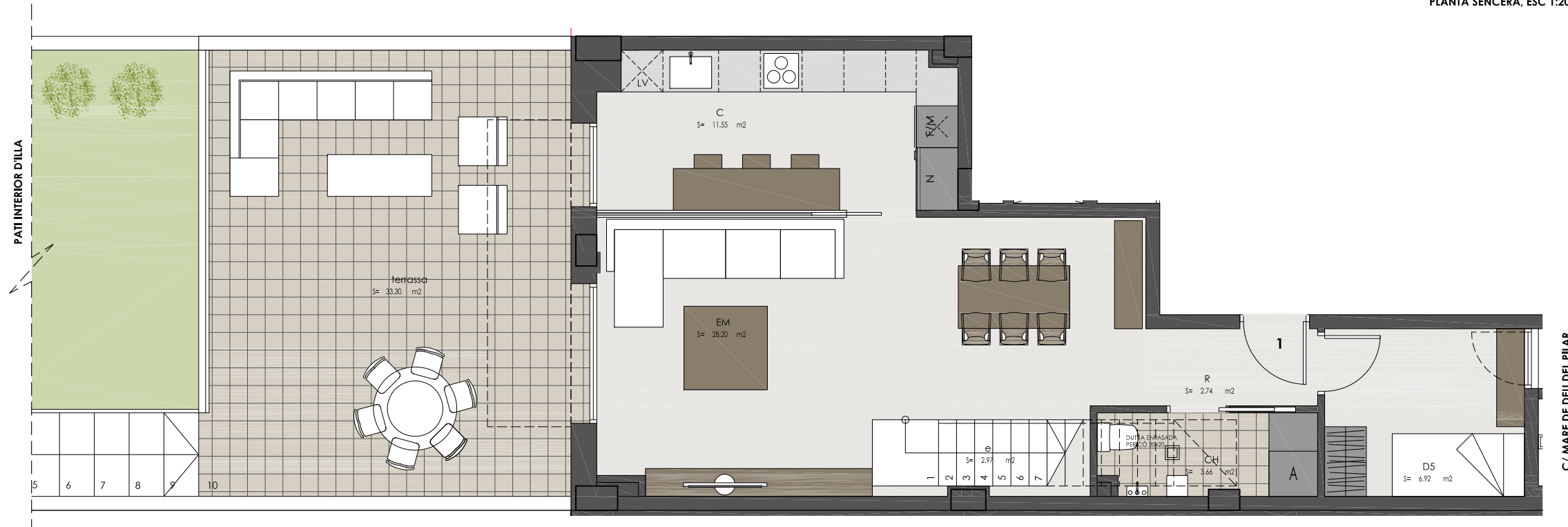
PLANTA SENCERA, ESC 1:200
