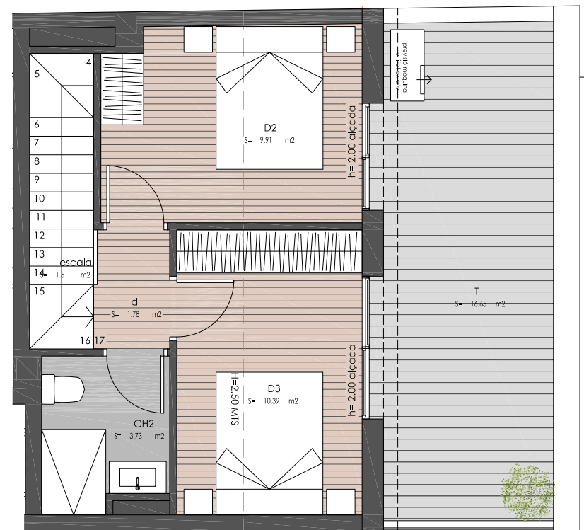
PLANTA SOTACOBERTA
