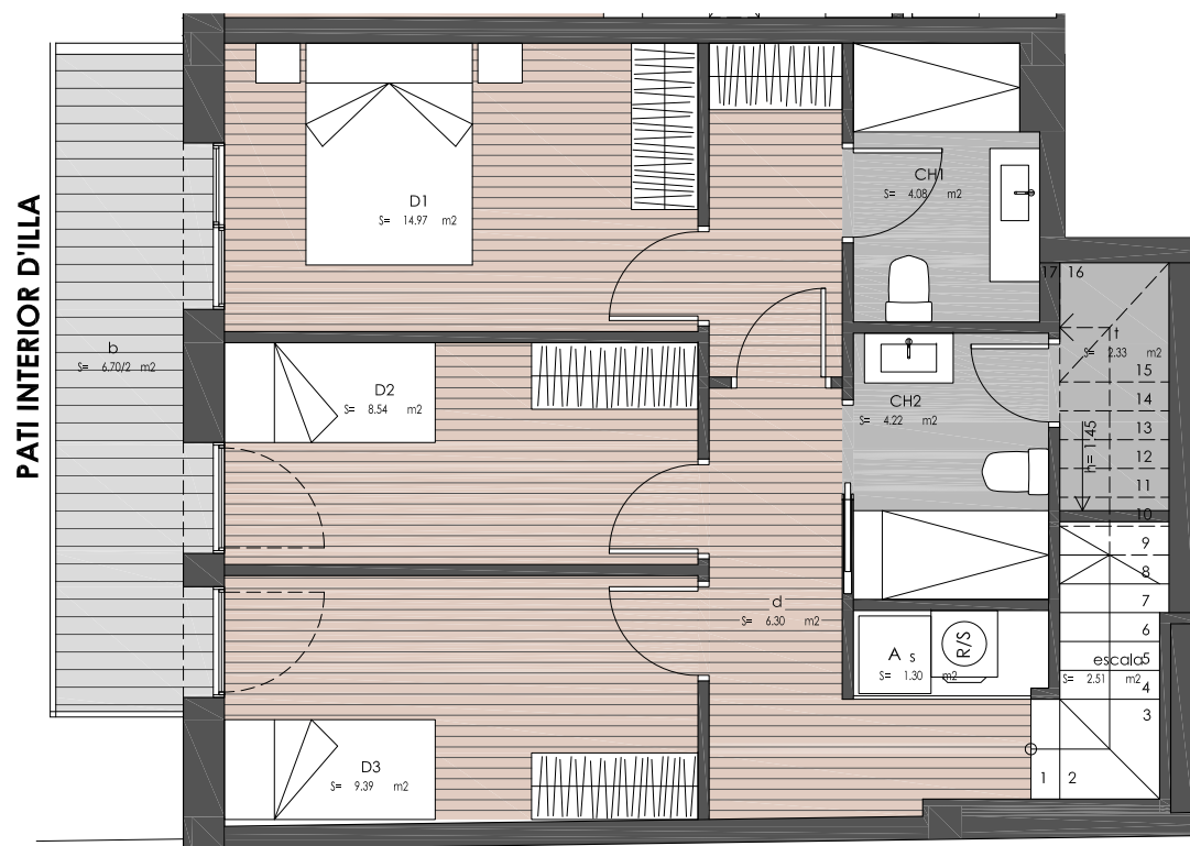
PLANTA TERCERA
