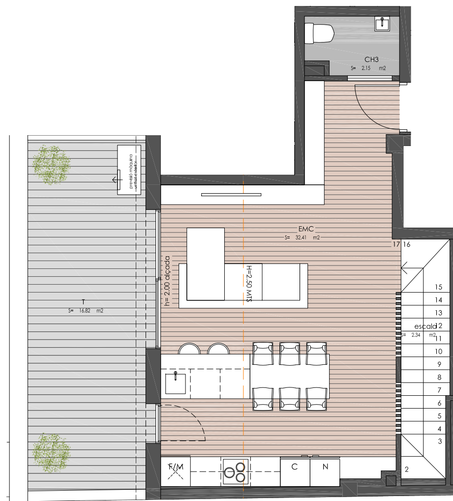
PLANTA SOTACOBERTA
